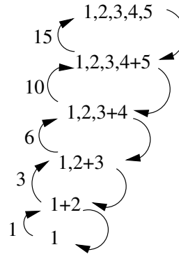
Figura 12.1: Árvores de recursão para m = 1 e n = 5 .
