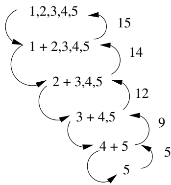
Figura 12.1: Árvores de recursão para m = 1 e n = 5 .
