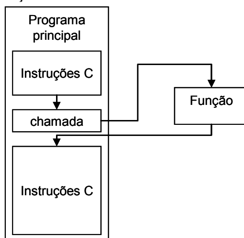
Figura 1 – Chamada de função e desvio de execução
