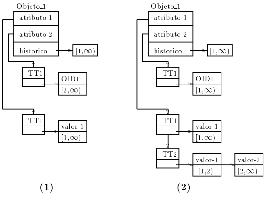
Figura 2: Os estados de Objeto_1 nos instantes TT1 e TT2 .
