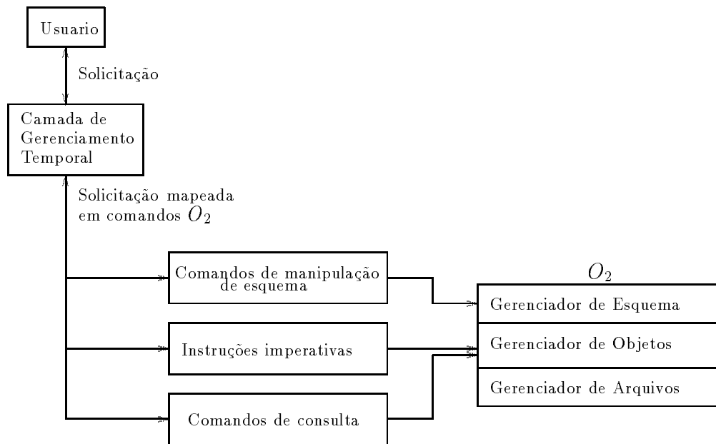
Figura 1: Processo de interação da Camada de Gerenciamento Temporal com o usuário e o O_2
