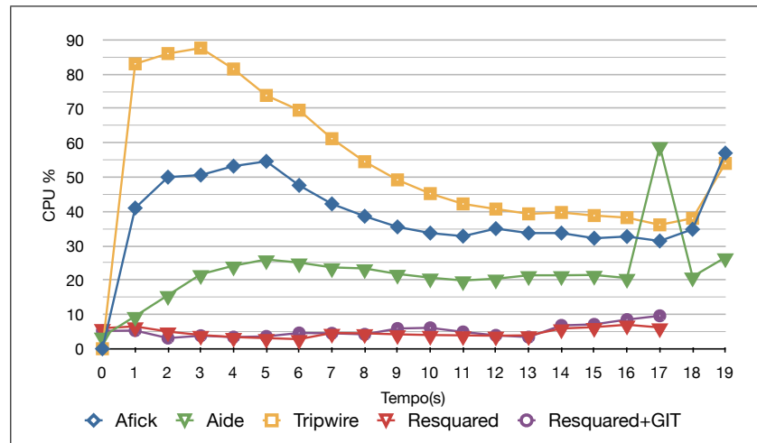
Figura 6.10: Porcentagem de CPU operação de verificação com diretório /usr/bin .
