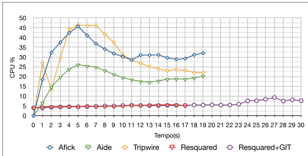
Figura 6.9: Porcentagem de CPU operação de inicialização com diretório /usr/bin .
