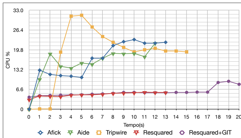
Figura 6.4: Porcentagem de CPU operação de inicialização com diretório /etc .
