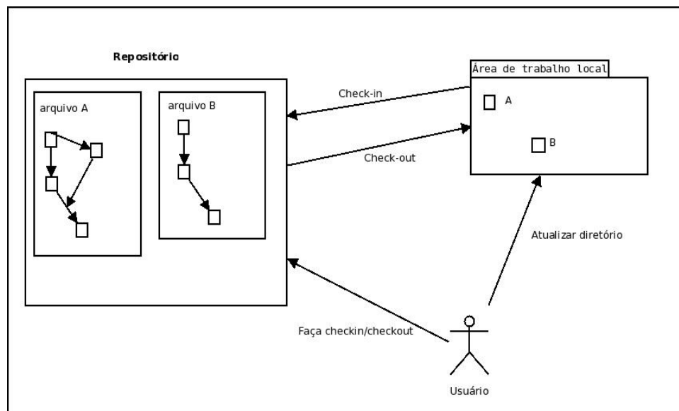
Figura 3.1: Exemplo do fluxo de dados do modelo check-in/check-out .
