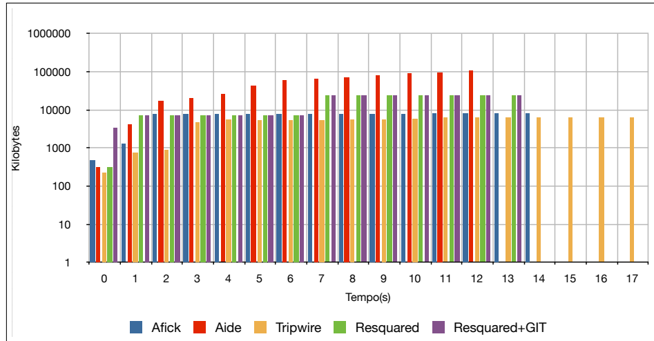
Figura 6.3: Consumo de memória da operação de verificação com diretório /etc .
