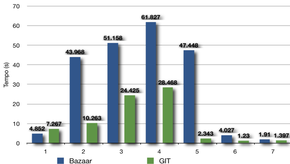
Figura 3.5: Comparativo de operações Mantha – Maio/2008.
