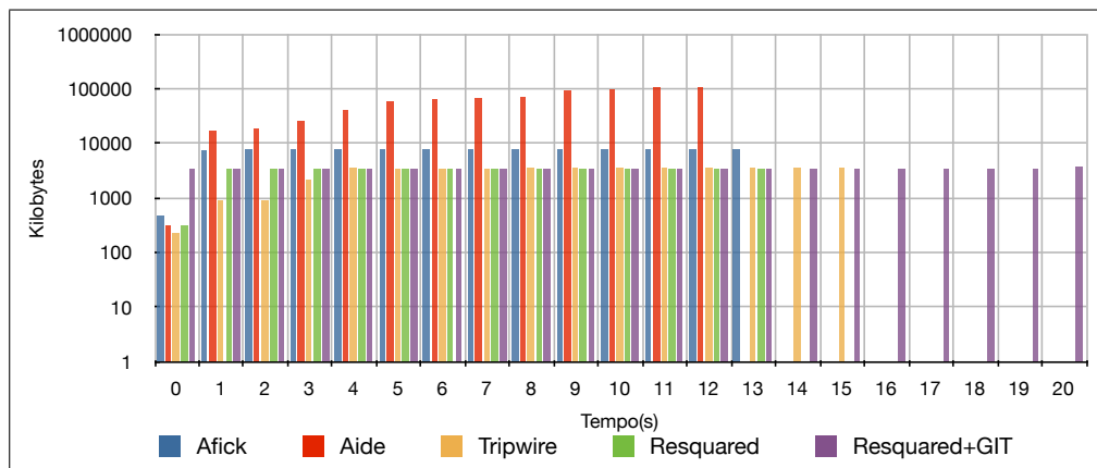
Figura 6.2: Consumo de memória da operação de inicialização com diretório /etc
