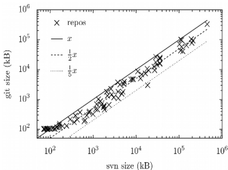
Figura 3.3: Comparativo dos tamanhos de repositório obtidos.
