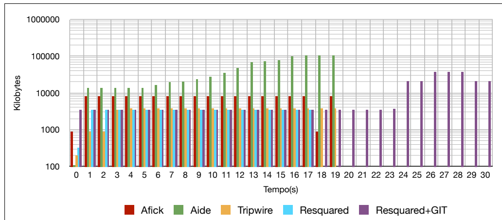
Figura 6.7: Consumo de memória da inicialização com o diretório /usr/bin .
