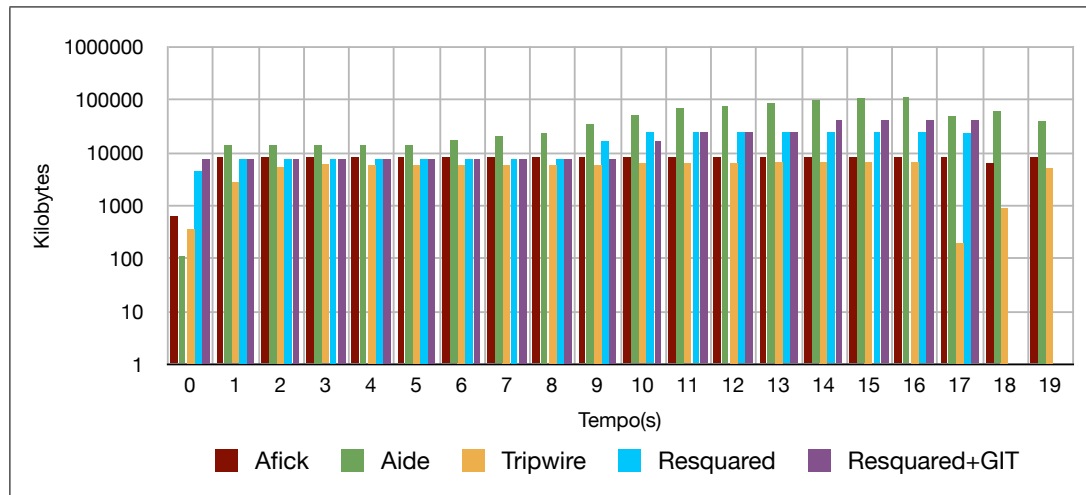
Figura 6.8: Consumo de memória da operação de verificação com o diretório /usr/bin .
