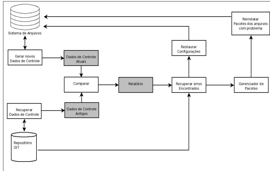
Figura 5.1: Diagrama de Fluxo Geral de Operação.
