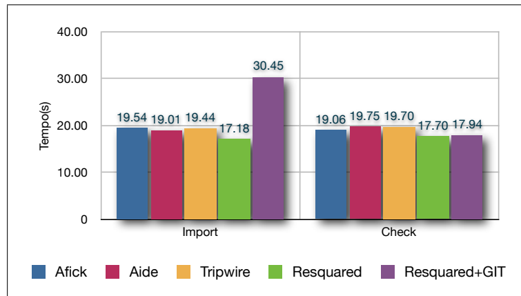
Figura 6.6: Tempo de execução sobre o diretório /usr/bin
