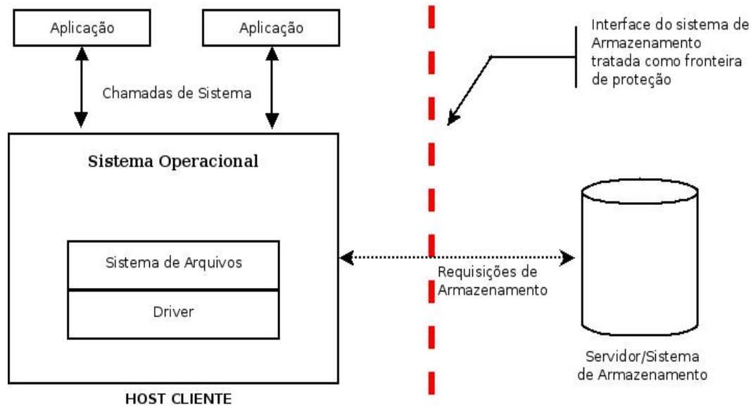
Figura 4.1: Esquema de storage-based IDS por Strunk et al. [52].
