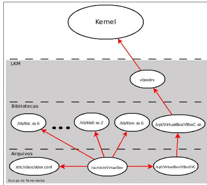
Figura 5.3: Exemplo de Árvore de execução do aplicativo VirtualBox.
