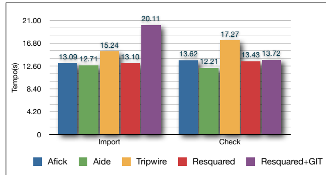
Figura 6.1: Tempo de execução sobre o diretório /etc
