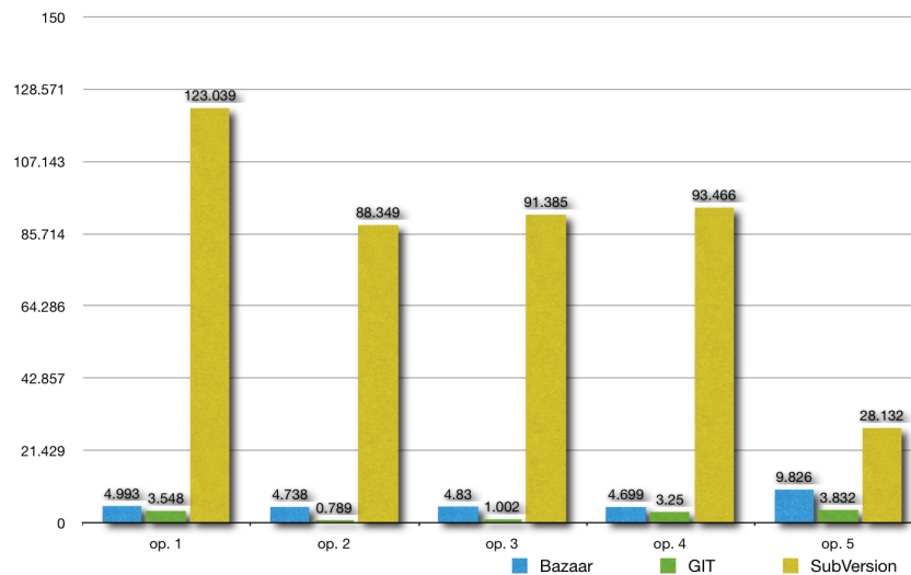
Figura 3.6: Comparativo de Operações sobre GIT, SVN e Bazaar.
