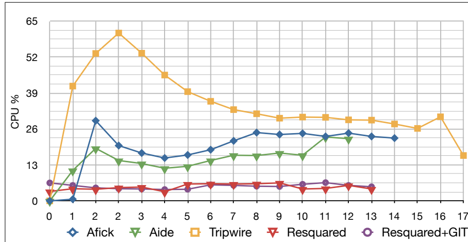
Figura 6.5: Porcentagem de CPU operação de verificação com diretório /etc .
