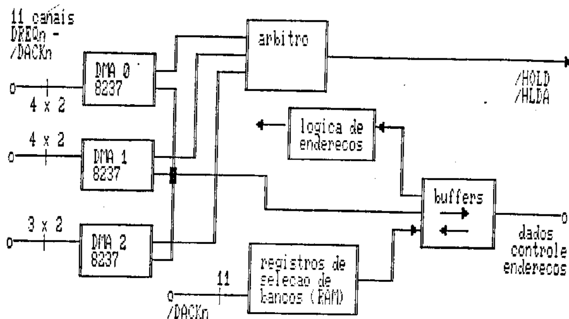
Figura 4.1 : arquitetura da placa controladora de DMA
