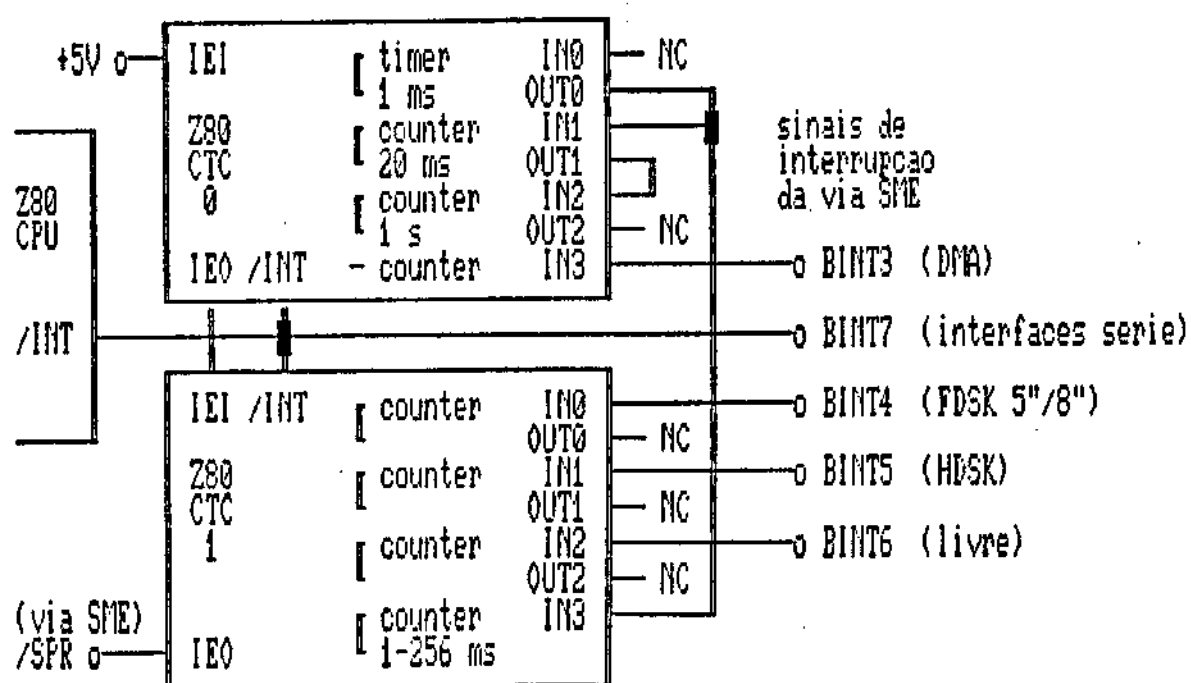
Figura 3.4 : estrutura padrão de temporizacao/interrupcao
