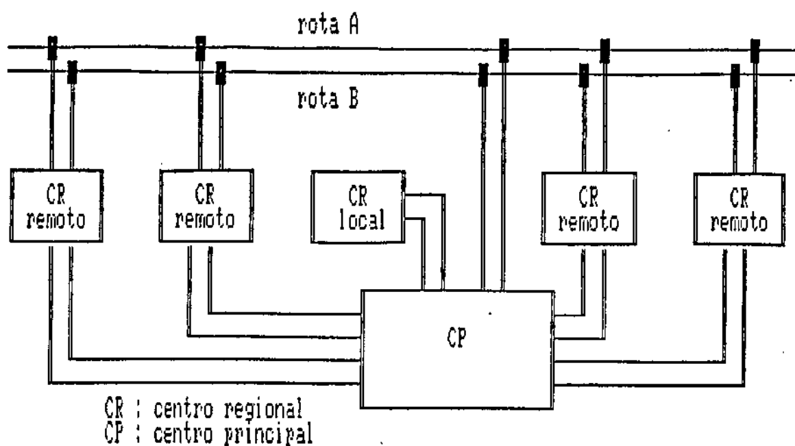
Figura 6.5 : arquitetura de comunicacao do sistema de telessupervisao
