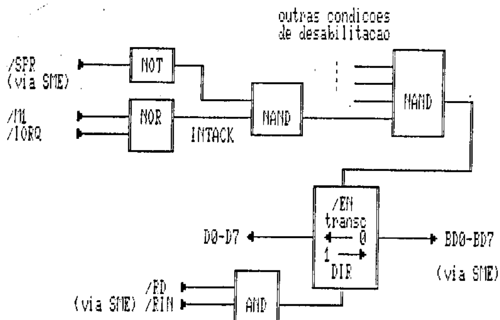
Figura 3.5 : logica de apoio a interrupções na placa de CPU
