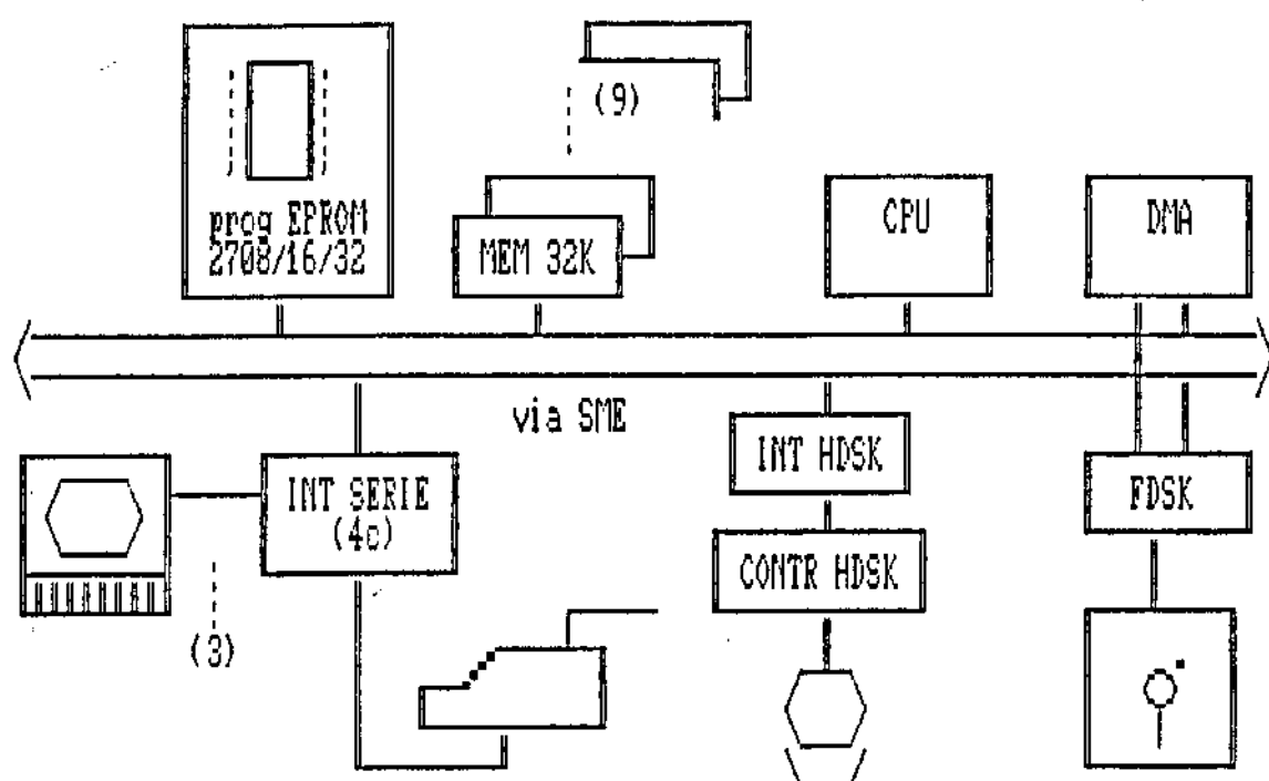
Figura 6.1 : configuracao do sistema multiusuario
