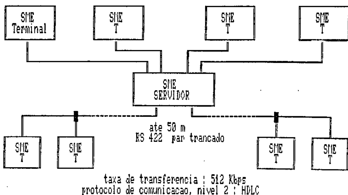
Figura 6.2 : arquitetura da rede servidor - terminais
