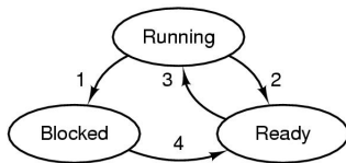
Tanenbaum: Figura 2.2
