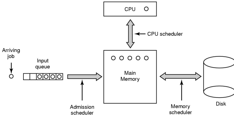
Tanenbaum: Figura 2.40
