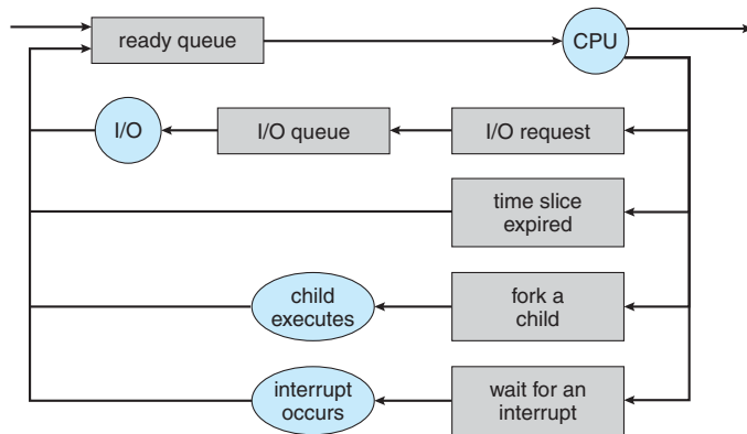
Silberschatz: Figura 3.06
