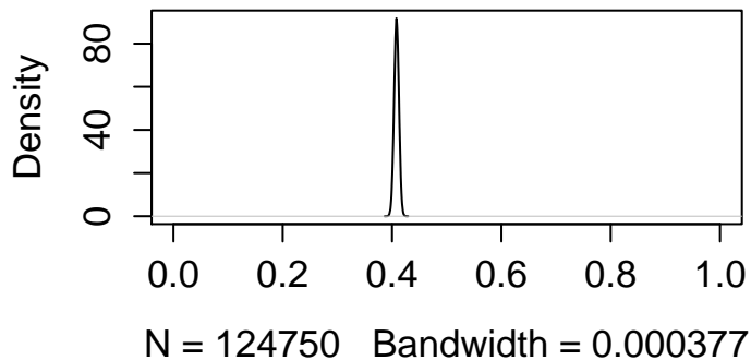
3000 dimensoes
