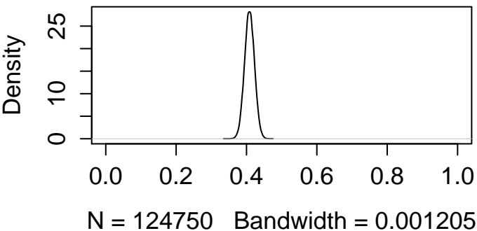
300 dimensoes
