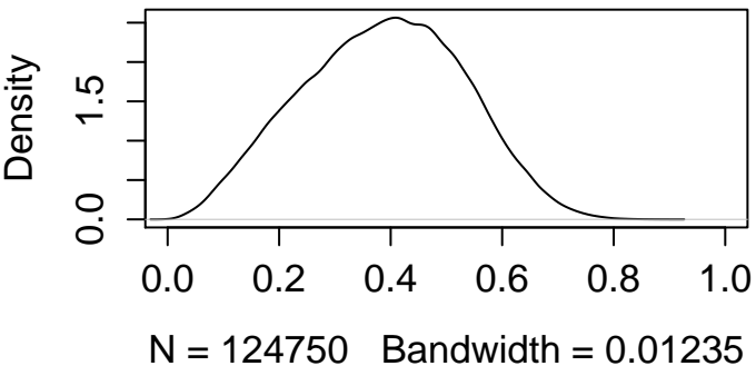
3 dimensoes
