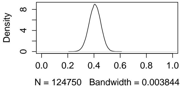
30 dimensoes
