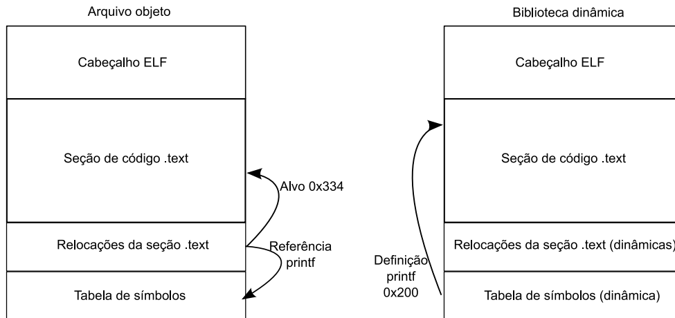
Figura 3: Ligando um objeto contra uma biblioteca dinâmica.
