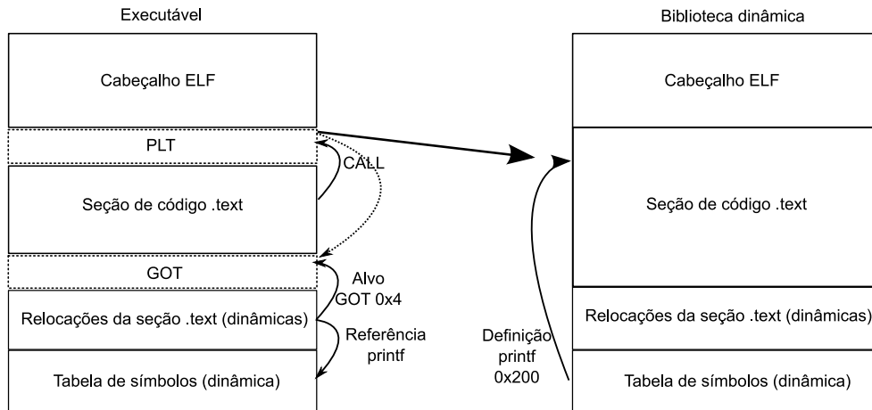
Figura 4: Ligação concretizada de um objeto contra uma biblioteca dinâmica.
