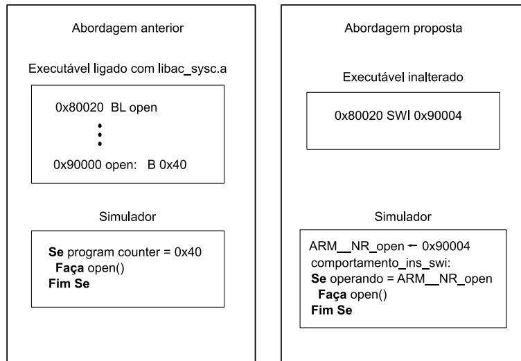
Figura 7: Esquematização comparando as duas abordagens para tratamento de chamadas de sistema no simulador ArchC.
