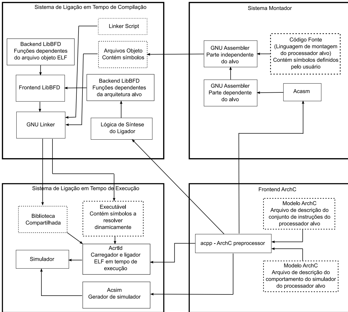
Figura 1: Diagrama da visão geral do sistema apresentado.
