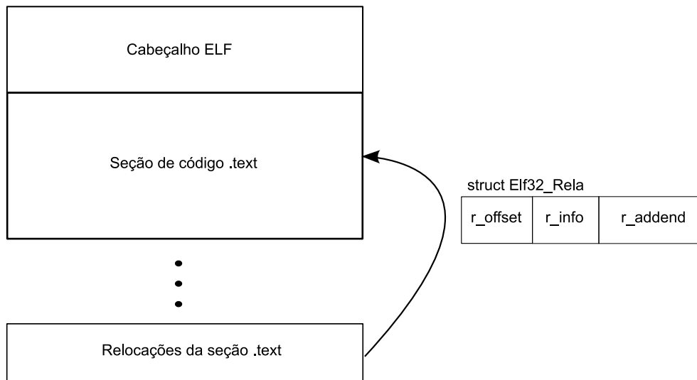
Figura 2: Relocações em um arquivo objeto ELF.
